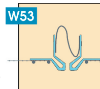
Dehnfugenprofil DUO-TEX Kratzputz
