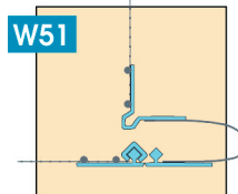
Dehnfugenprofil DUO-TEX Ecke
