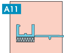
Anputzleiste MINI
