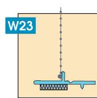
Gewebeleiste STANDARD-UV
