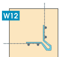
Gewebeeckwinkel DUOTEX Kratzputz
