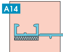
Anputzleiste UNIVERSAL
