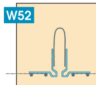
Dehnfugenprofil DUO-TEX Fläche
