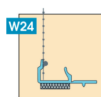
Gewebeleiste IDEAL
